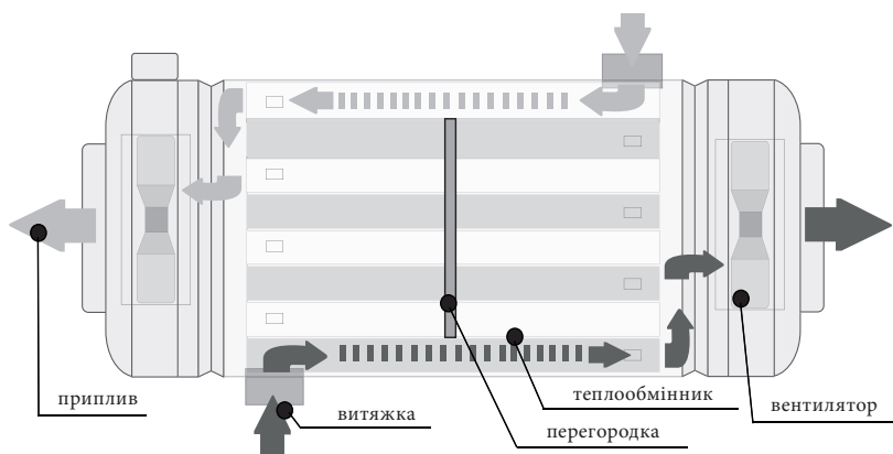
Рис. 1а. Схема повітряних потоків для систем типу «AB» з центральним притоком і 2-канальною симетричною витяжкою (вільна установка).
