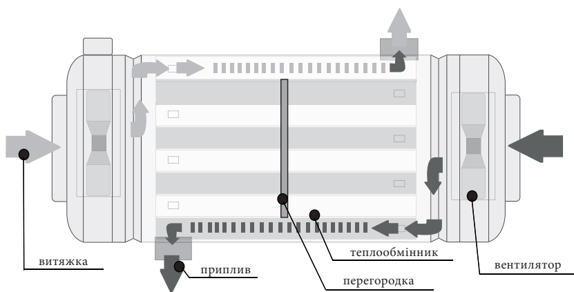
Рис. 1б. Схема повітряних потоків для систем типу «BB» (виготовляється під замовлення) з центральною витяжкою і 2-канальним симетричним притоком (вільна установка).
