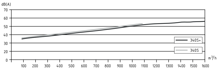
Рис. 5. Загальний рівень звукового тиску вентиляційних систем PRANA-340S і PRANA-340S+ на відстані 3 метри в режимі «рекуперація», дБ(A).
